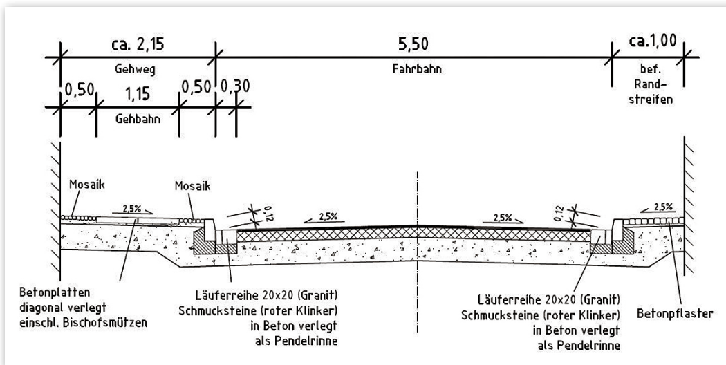
Eine mögliche Variante für den Querschnitt der sanierten Buchtstraße. Quelle: Redeker Consult Luckenwalde
